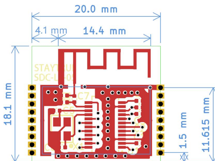
模组尺寸图
